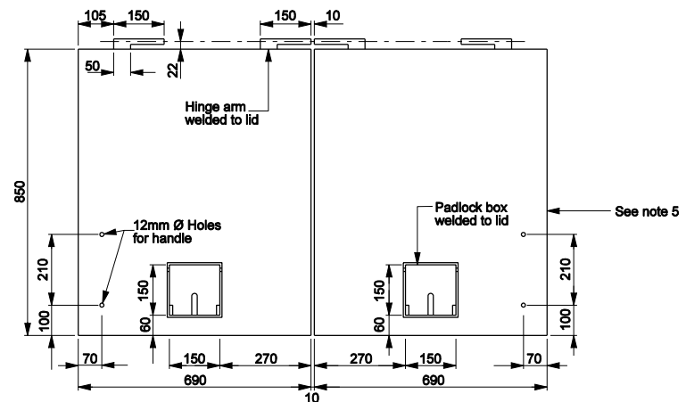
DOUBLE LID (3085 & 3102 Pumps)
