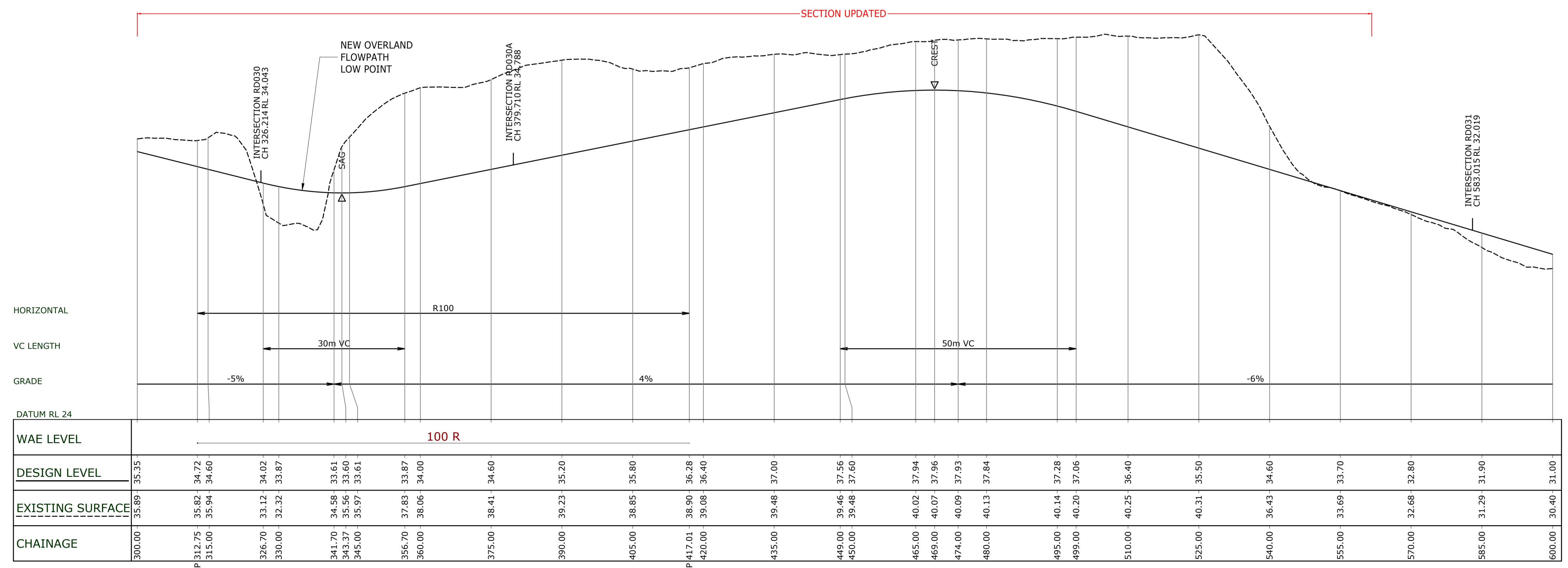
RD004 LONGITUDINAL SECTION 1:500 HORI. 1:100 VERT.
